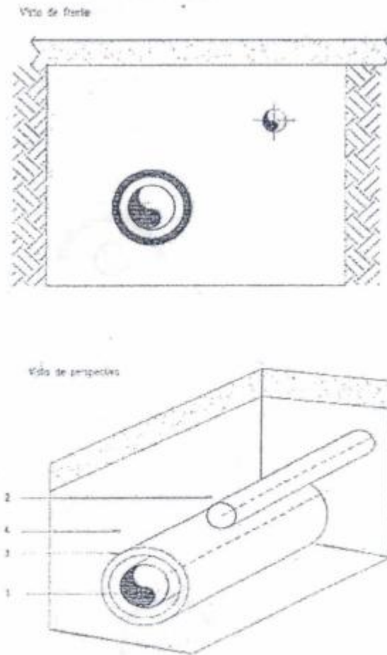
Figura 7a Protección con encamisado continuo de PE/PVC/PP/PRFV Paralelismo
