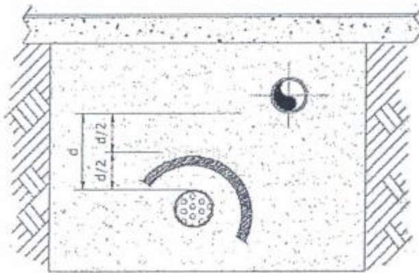
Figura 6a Protección con media caña o media caña de PE/PVC/PP/PRFV más placas de caucho sintético Paralelismo
